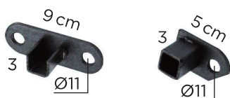
Platine haute et basse
